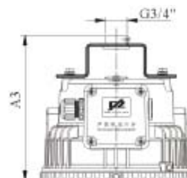
Pendant Bracket
